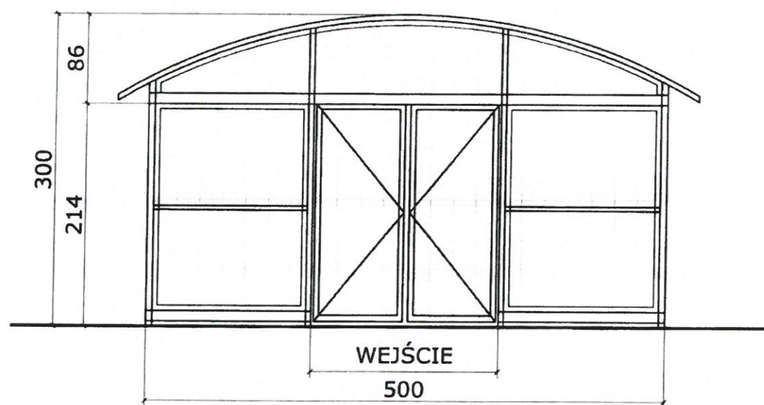
ELEWACJA WSCHODNIA
