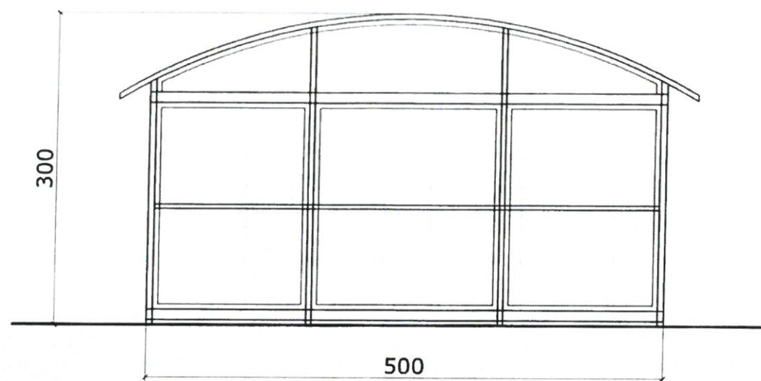
ELEWACJA ZACHODNIA
