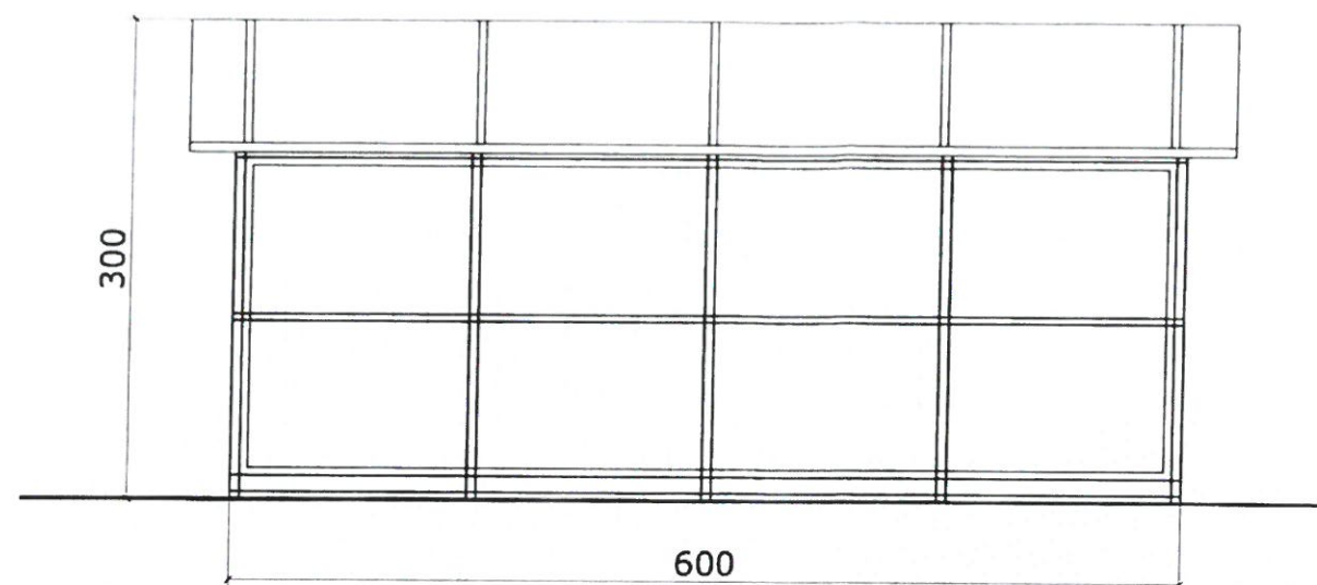
ELEWACJA PÓŁNOCNA
